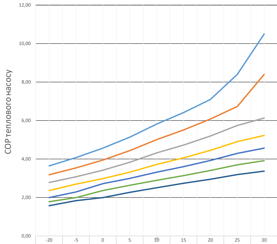
ГРАФІК COP МОНОБЛОК RAY-15MN RAYMER залежність температури навколишнього середовища та температури гарячої води на виході, фреон R410A
